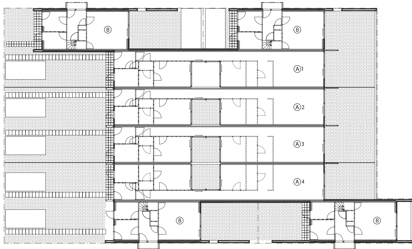
PLATTEGRONDEN TYPE A & B
